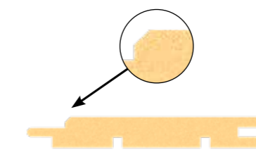
1. SAUNA-WANDVERKLEIDUNG MIT STP-PROFIL
