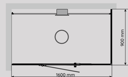
VISTA 160 RECHTS Maße: T 900 x B 1600 mm
